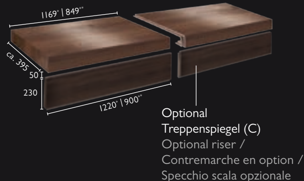
Typ 2B Treppenstufe mit Nase + Seitenabschluss Step with flange + side edge / Escalier avec nez de marche / Gradino con naso + terminale laterale
