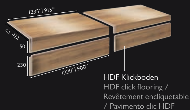
Typ 1A Treppenstufe Klassik Classic stair / Marche classique / Gradino classico
