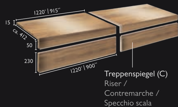
Typ 1B Treppenstufe Klassik + Seitenabschluss Classic stair + side edge / Marches d'escalier à finition latérale / Gradino classico + terminale laterale
